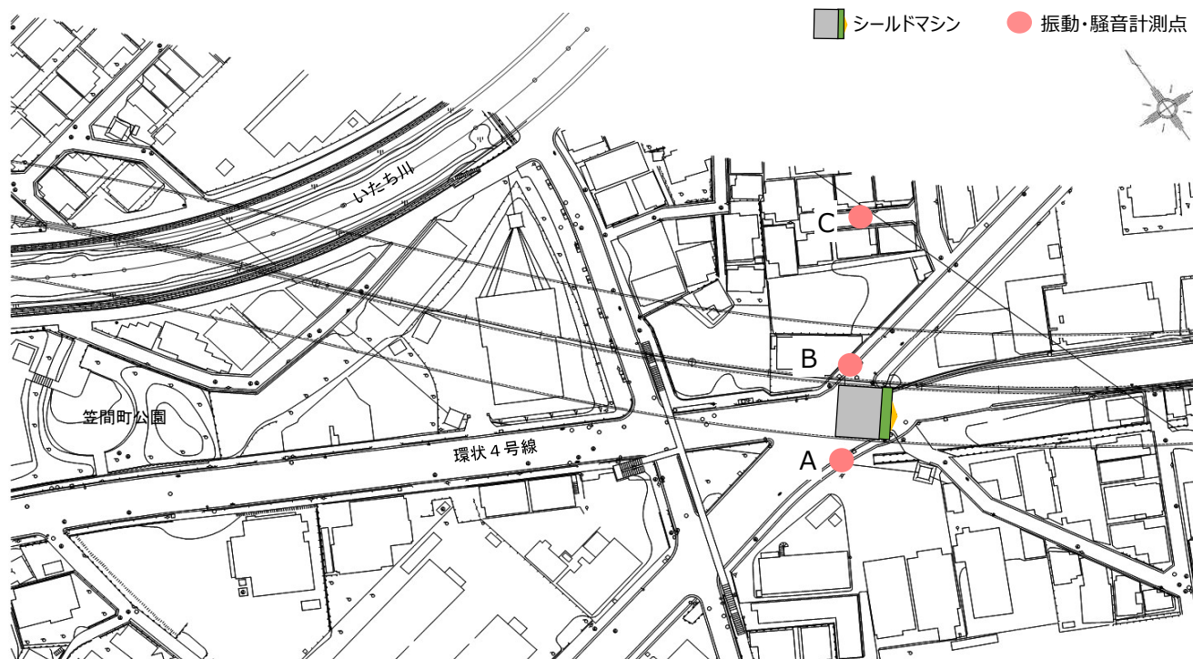
【シールドマシン位置図（11月2日時点）】
