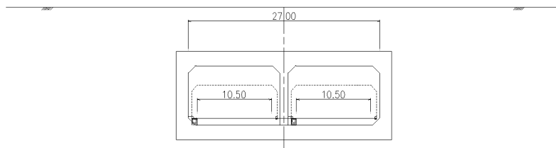
図 2-6 横断面図（地下式（トンネル部Ⅰ））
