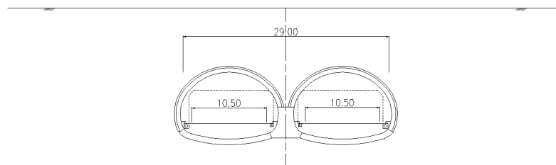
図 2-7 横断面図（地下式（トンネル部Ⅱ））
