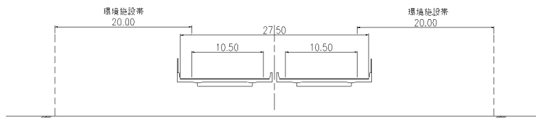
図 2-3 横断面図（嵩上式（橋梁部））
