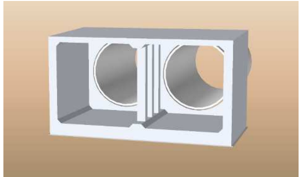
立坑部
