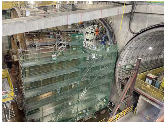
シールドマシン解体（R8.6撮影）
