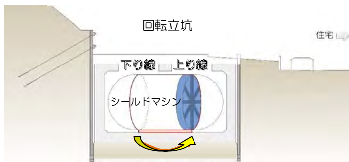
シールド機回転イメージ
