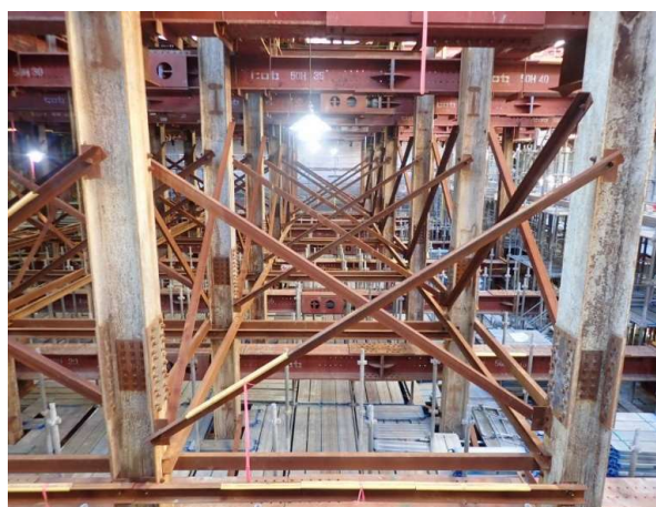
立坑内写真（側壁構築状況） R3.12.13撮影
