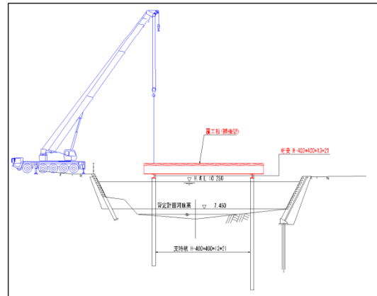
②覆工板を設置します
