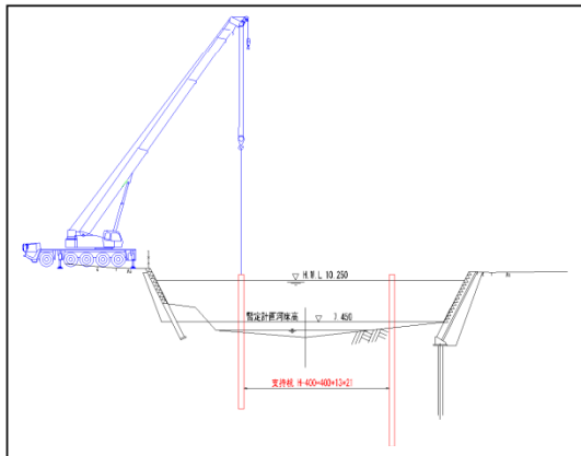
①杭を打ち込みます
