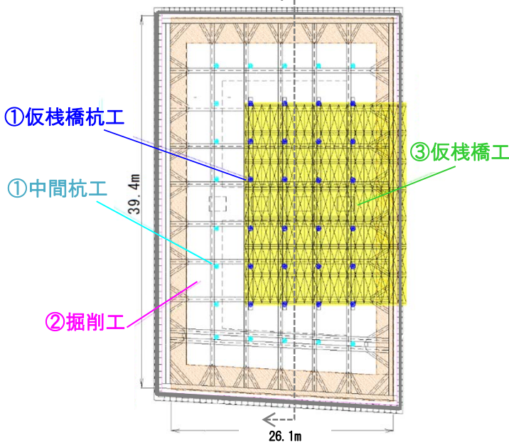
平面図
